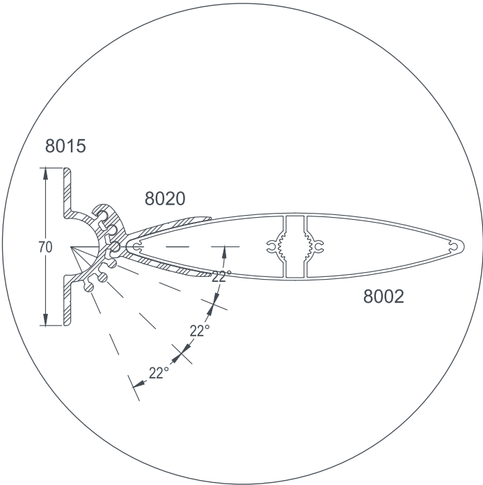
DETAY
