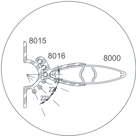
DETAY
