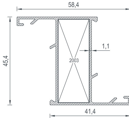
2029 BİRİM AĞIRLIK - Weight 0,597 (kg/mt)
