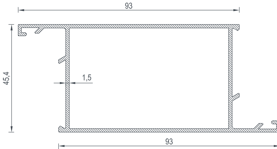
2023 BİRİM AĞIRLIK - Weight 1,196 (kg/mt)
