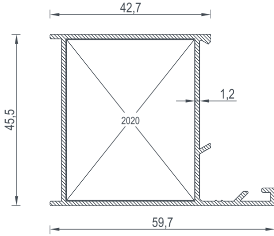
2006 BİRİM AĞIRLIK - Weight 0,662 (kg/mt)
