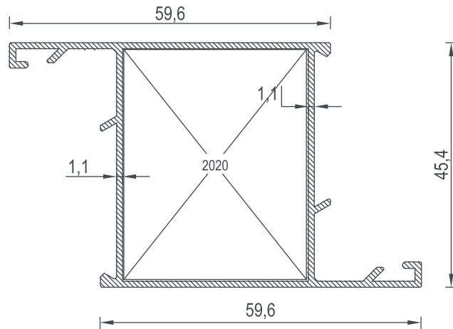
2037 BİRİM AĞIRLIK - Weight 0,710 (kg/mt)
