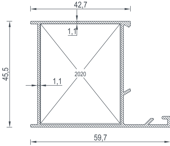
2039 BİRİM AĞIRLIK - Weight 0,614 (kg/mt)
