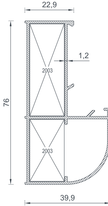
1937 BİRİM AĞIRLIK - Weight 0,834 (kg/mt)
