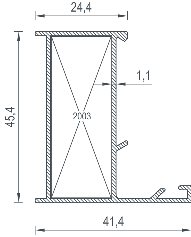
2030 BİRİM AĞIRLIK - Weight 0,500 (kg/mt)
