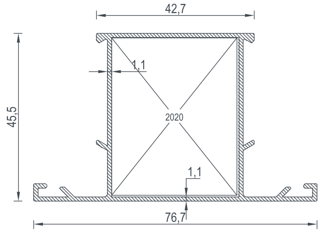
2038 BİRİM AĞIRLIK - Weight 0,713 (kg/mt)
