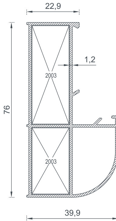
1941 BİRİM AĞIRLIK - Weight 0,913 (kg/mt)
